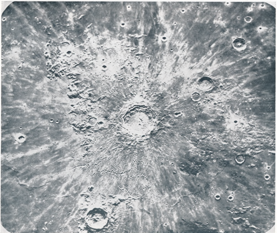
FIG. 2.—Crater Copernicus.
